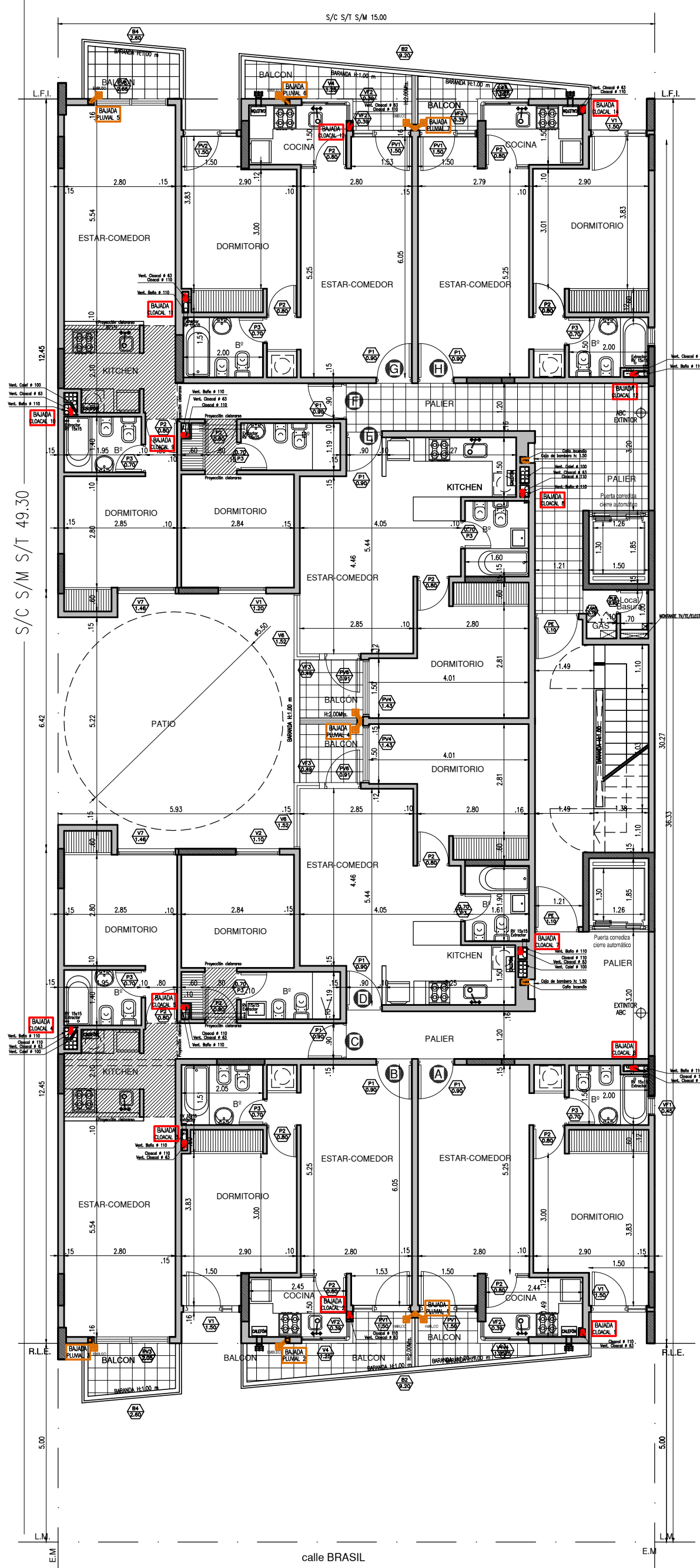
PLANTA 3° - 6°
