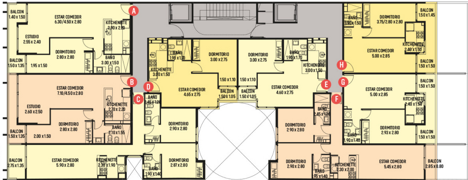
PLANTA TIPO 2º A 6º PISO
