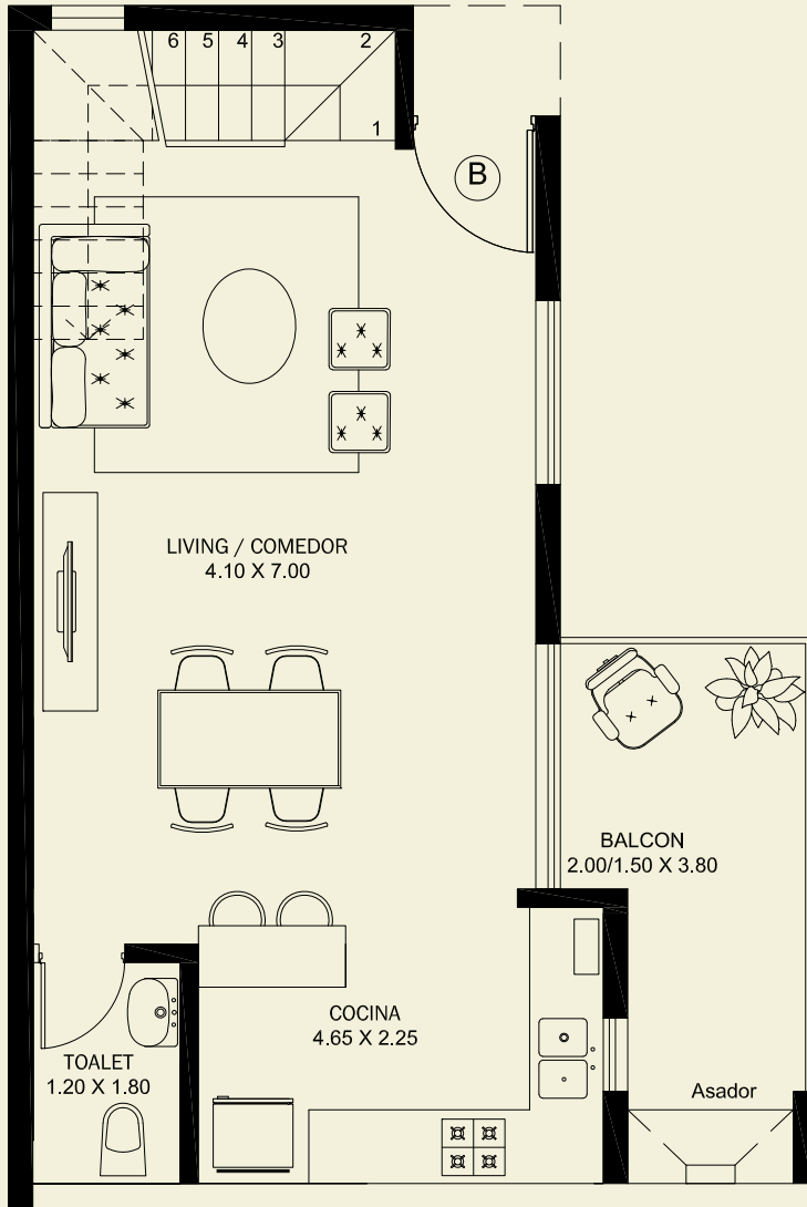
PLANTA BAJA
